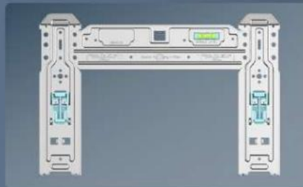
Kovový panel s vodováhou
